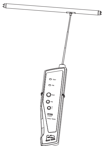
UT651B灯管测试示意图(图五)
