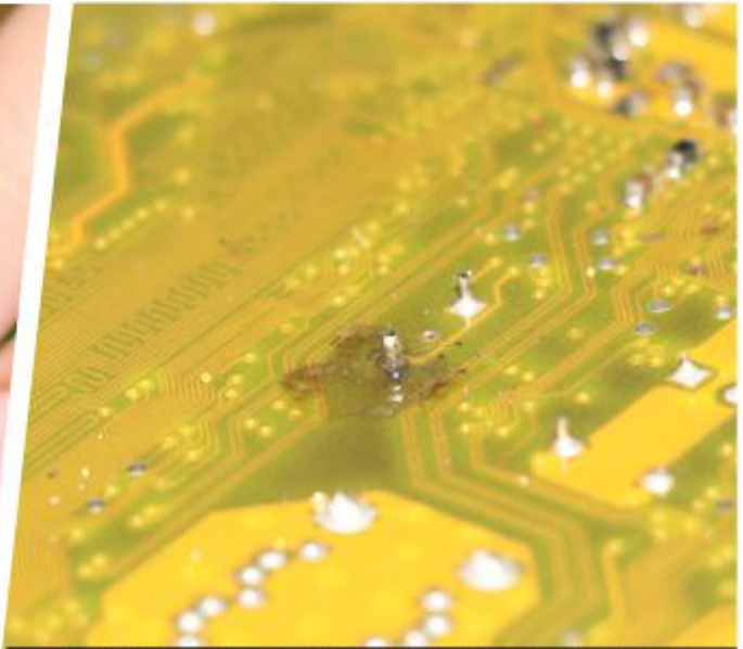
焊锡融化后即被吸锡线吸取
