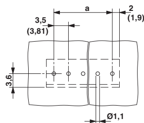
钻孔图
