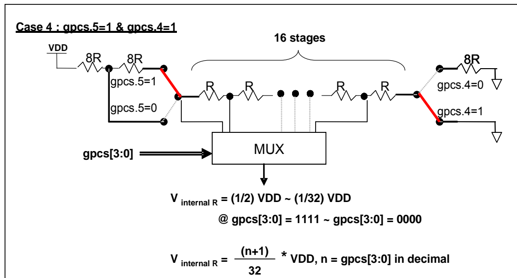
图 23 V_{\text{internal R}} 硬件接法 (gpcs.5=1 & gpcs.4=1)
