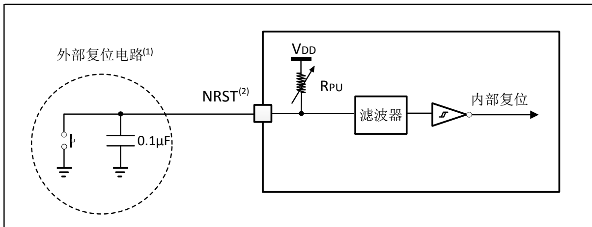
图 16. 建议的 NRST 引脚保护
