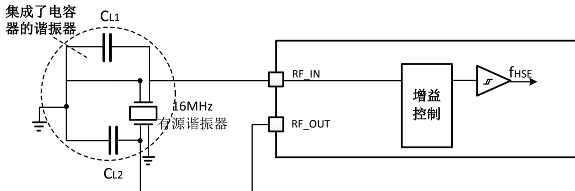
图11. 射频模块使用16MHz晶体的典型应用
