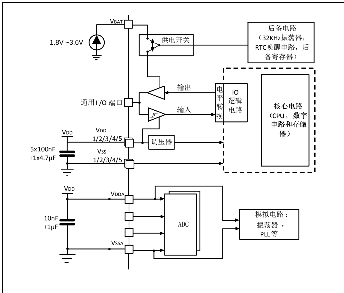
图 7. 供电方案
