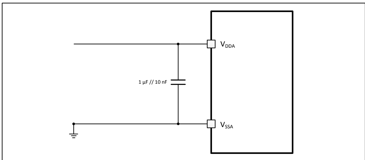
图24. 供电电源和参考电源去藕线路
