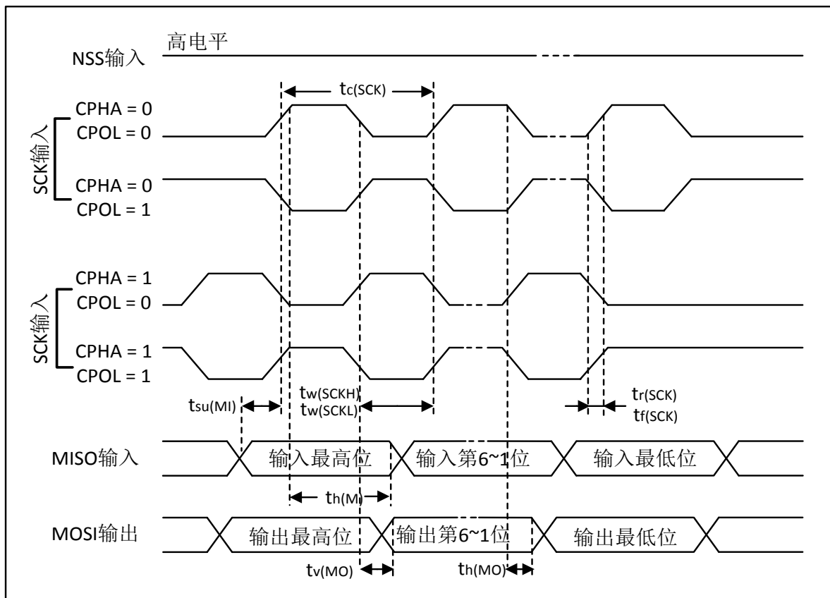
图 20. SPI 时序图-主模式 (1)
