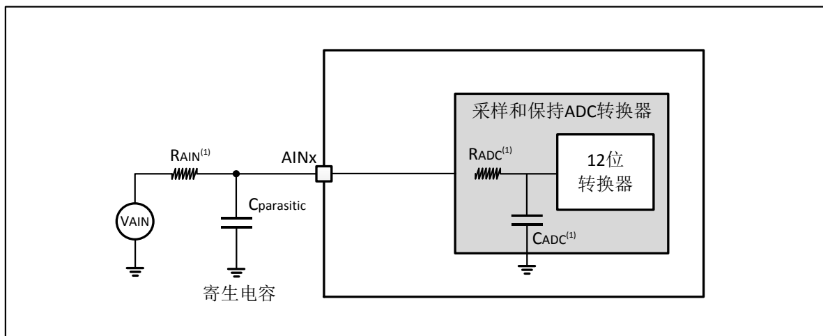
图22. 使用ADC典型的连接图
