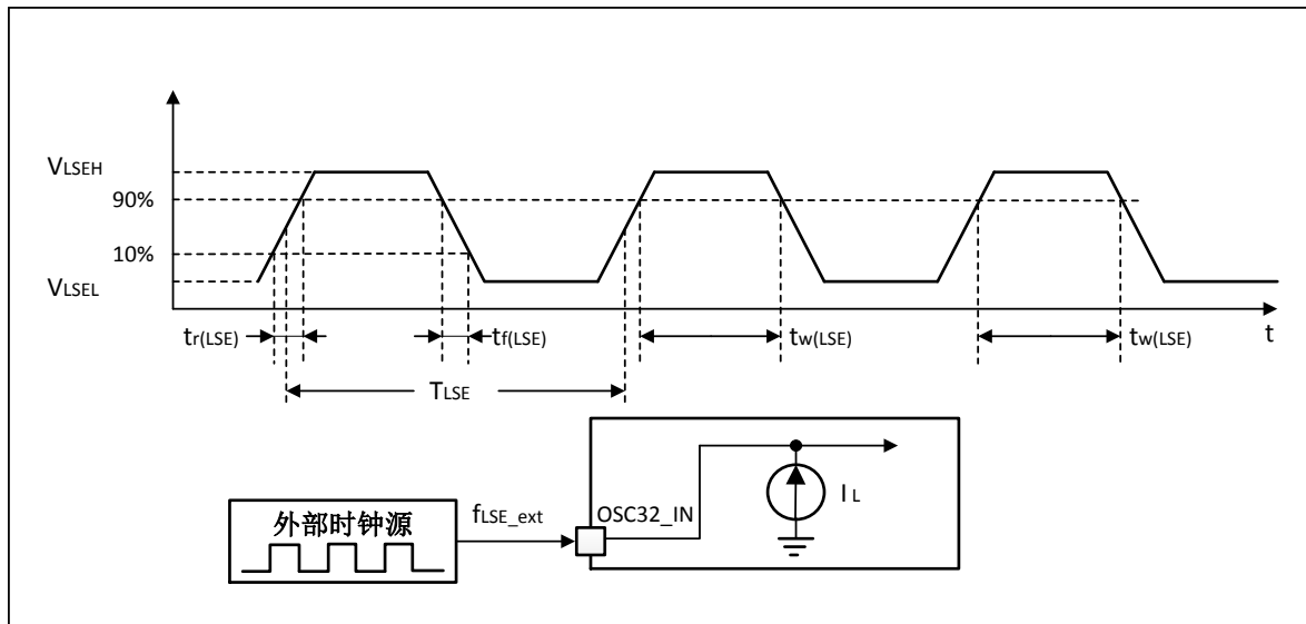
图 13. 外部低速时钟源的交流时序图
