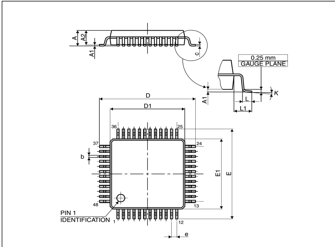
图 27. LQFP48, 48 脚低剖面方形扁平封装图
