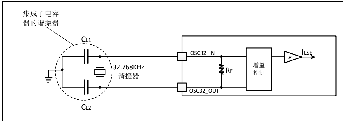
图 14. 使用 32.768KHz 晶体的典型应用
