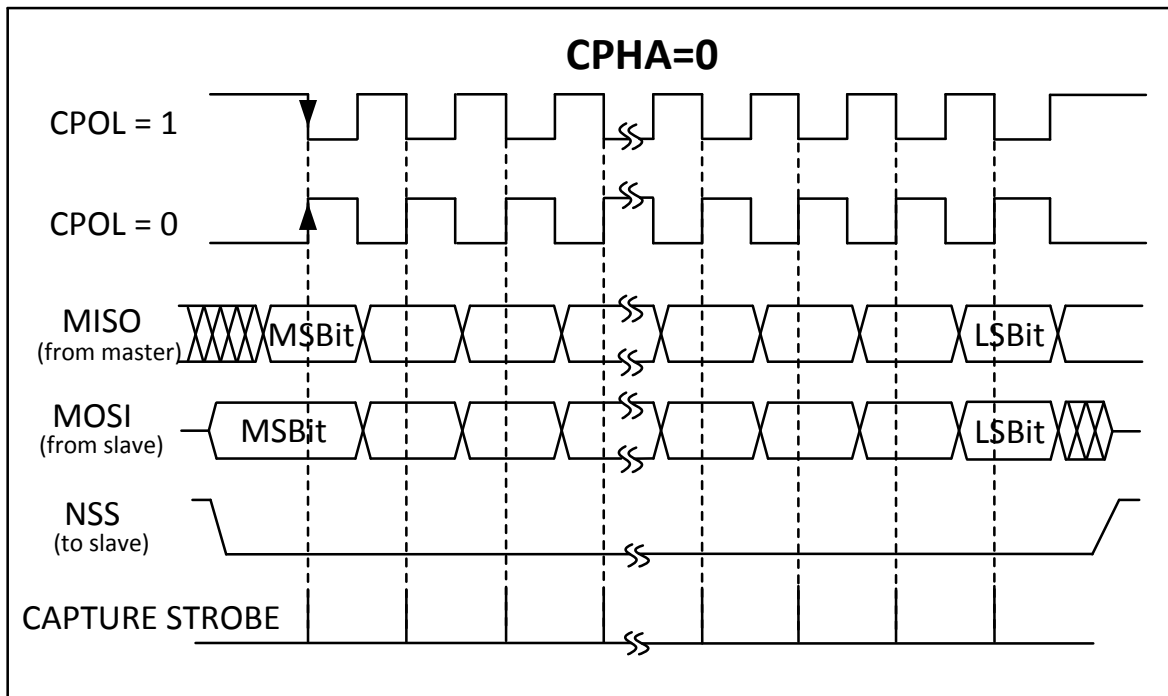
图 18. SPI 时序图-从模式和 CPHA = 0
