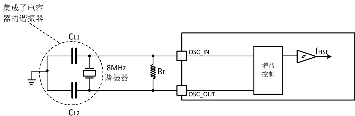
图10. 控制模块使用8 ~ 24MHz晶体的典型应用
