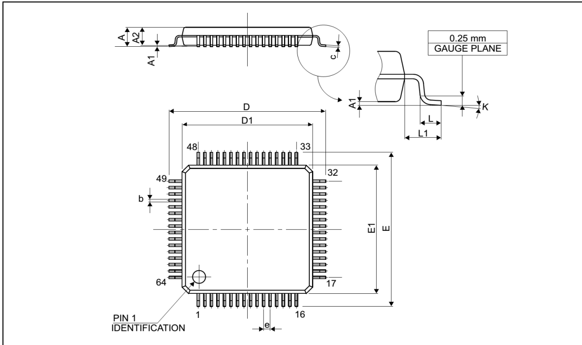
图 26. LQFP64, 64 脚低剖面方形扁平封装图
