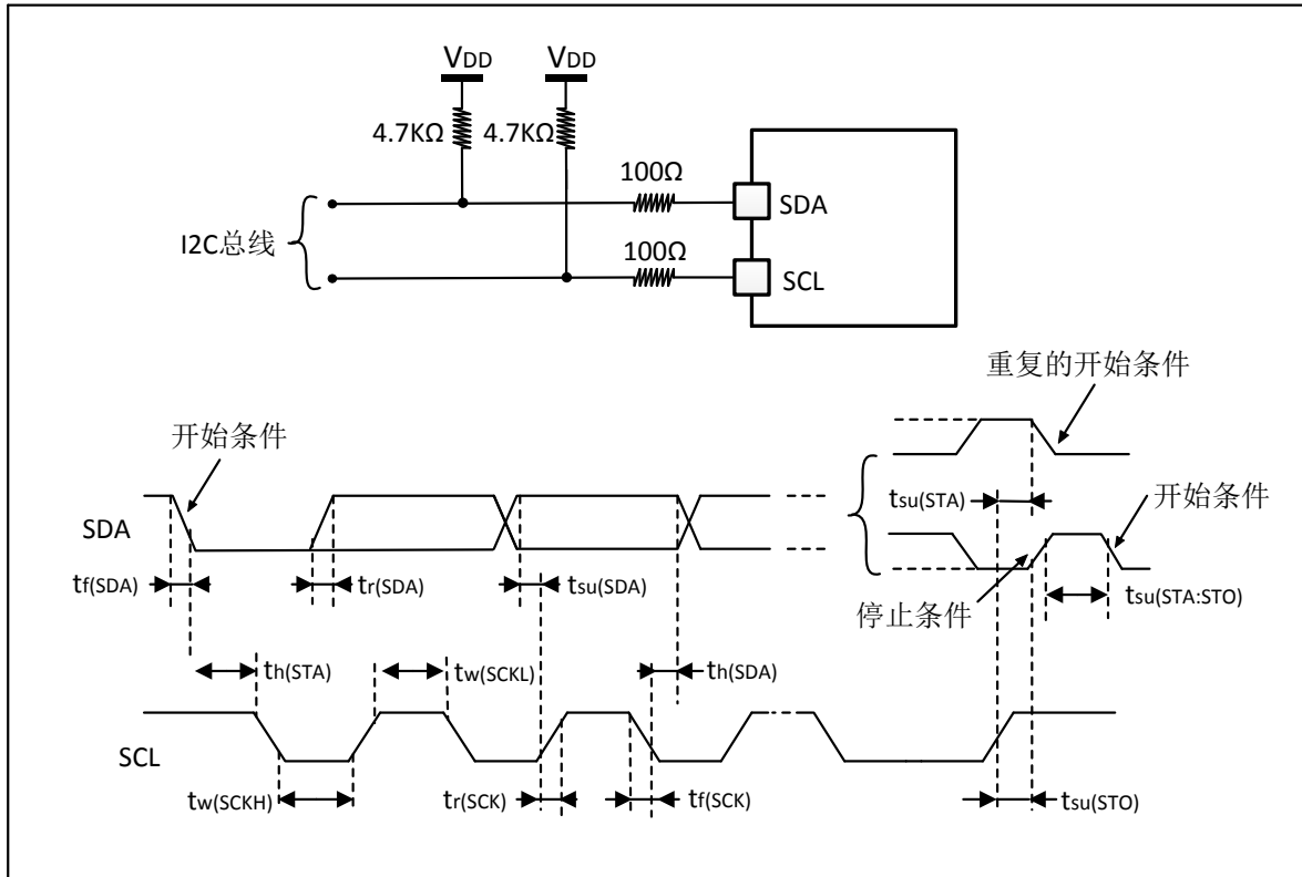
图 17. I 2 C 总线交流波形和测量电路 (1)
