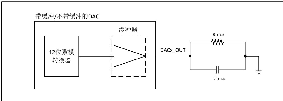
图23. 12Bit带缓冲/不带缓冲DAC
