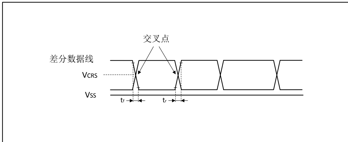
图 21. USB 时序：数据信号上升和下降时间定义
