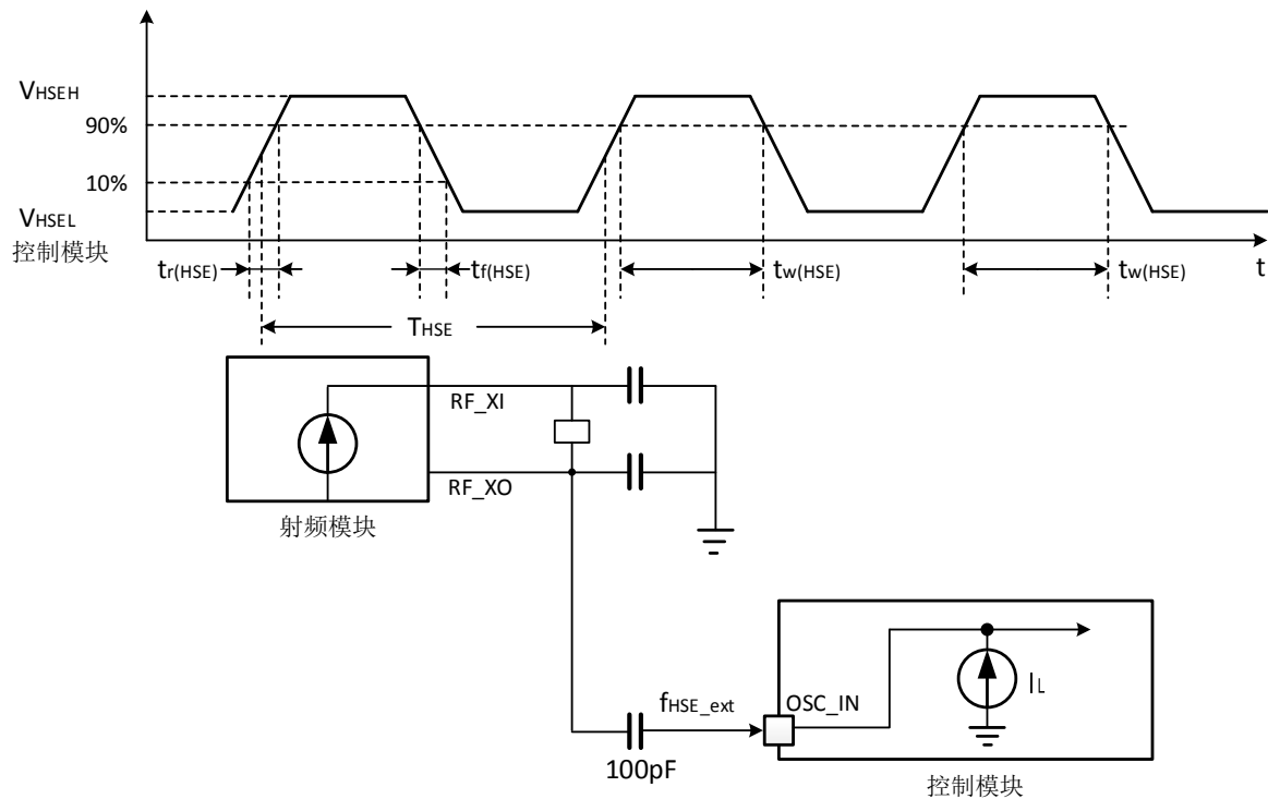
图12. 外部高速时钟源的交流时序图
