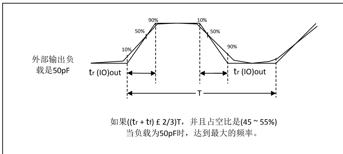
图 15. 输入输出交流特性定义
