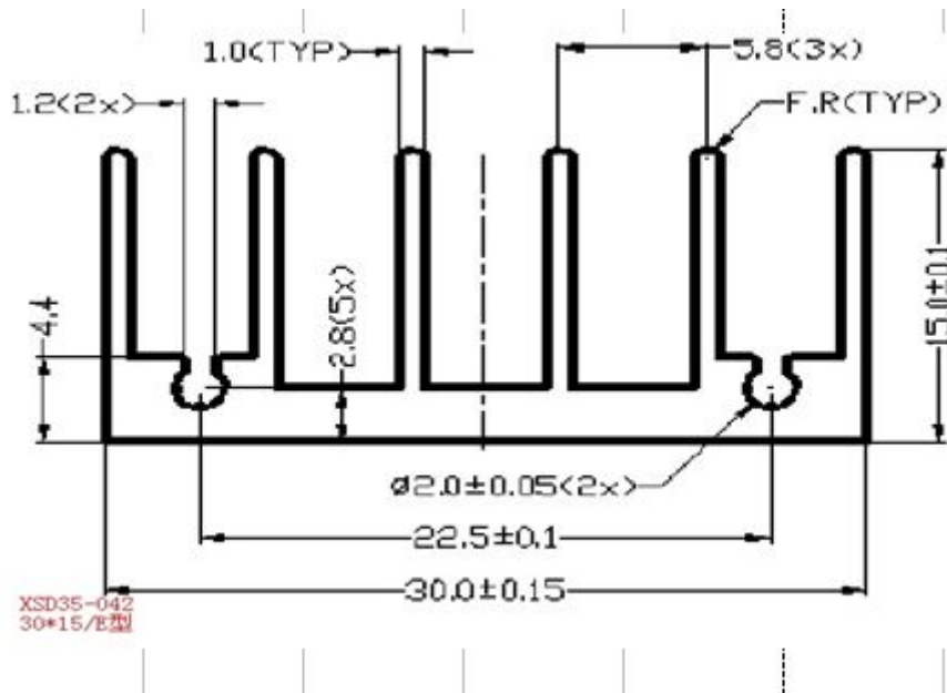
产品尺寸图
