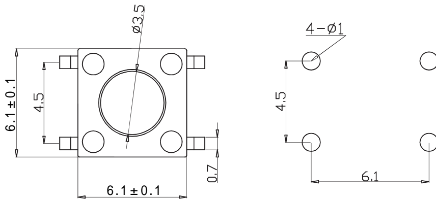
安装尺寸
