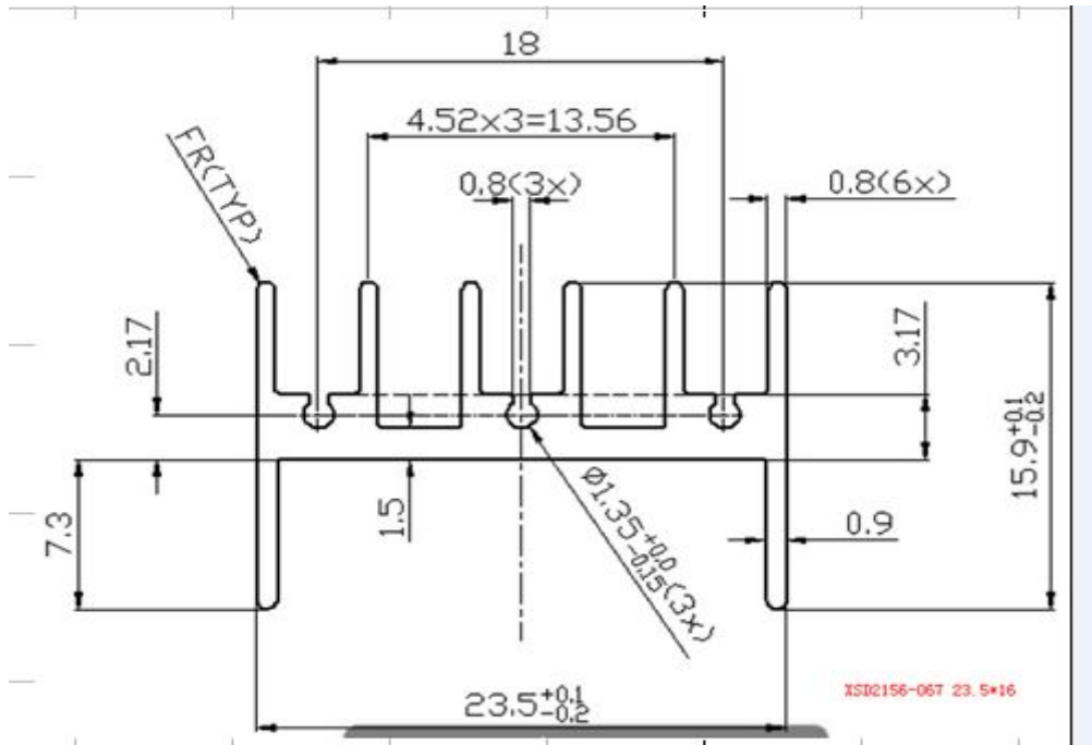
产品尺寸图
