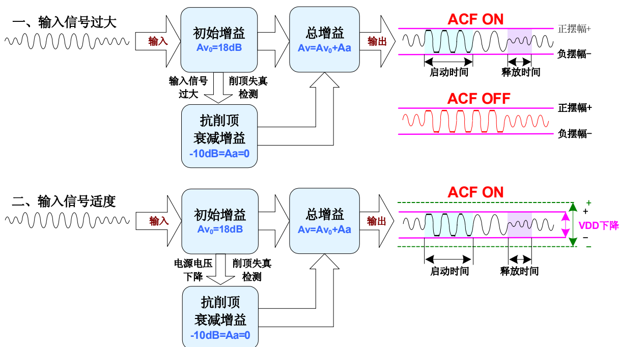
图 2 ACF 工作原理示意图
