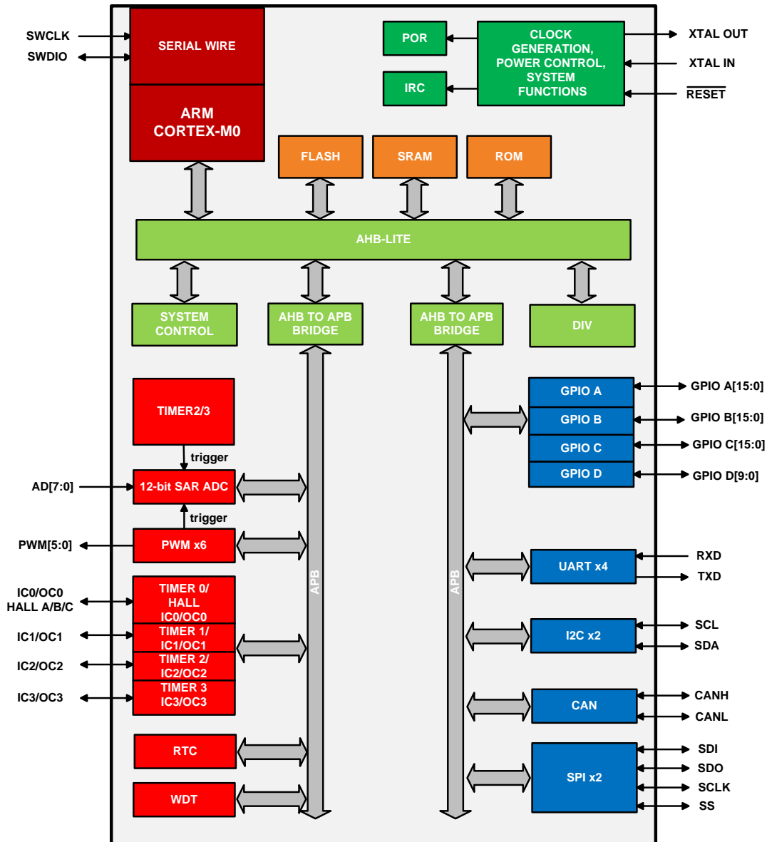
图 4-1 功能方框图
