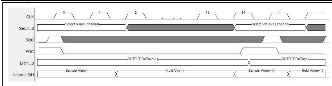
图 6-40 SAR ADC 连续采样示意图
