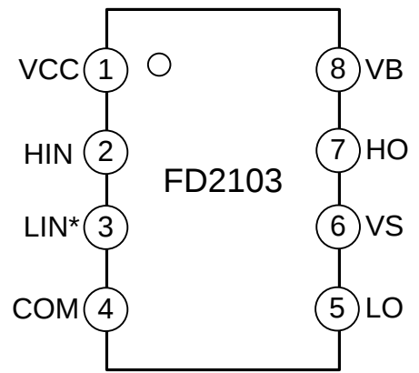
图 6-1 封装管脚图
