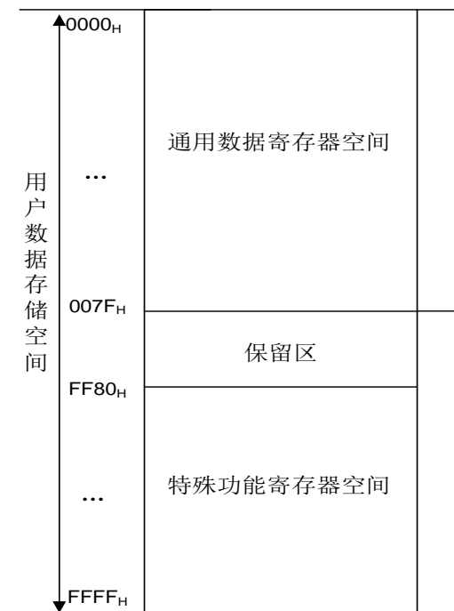
图 3-2 数据区地址映射示意图
