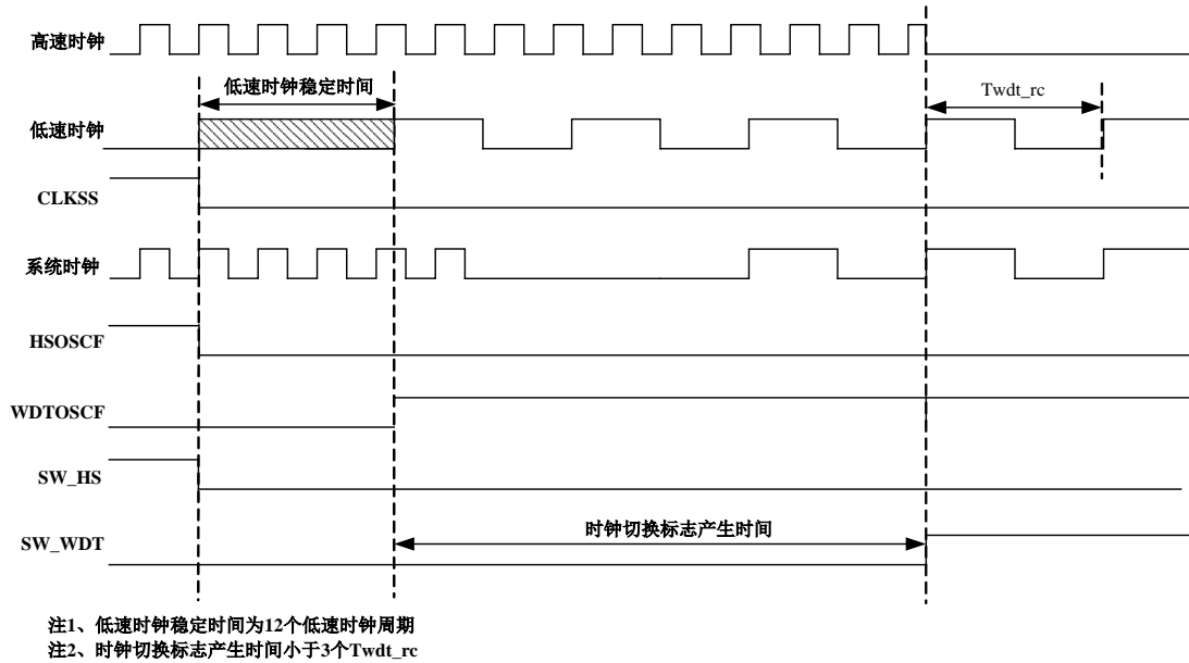
图 6-4 INTOSCH/HS/XT 时钟切换到 INTOSCL 时钟
