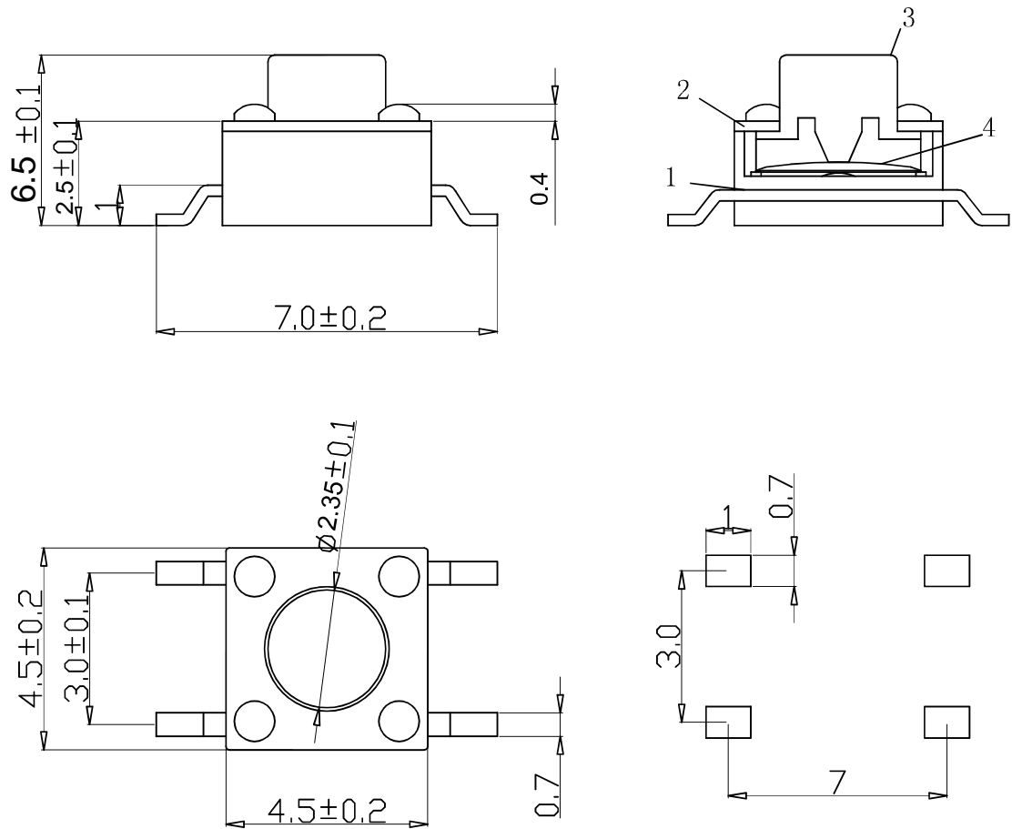
安装尺寸
