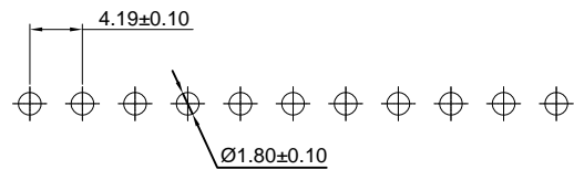
P.C.B LAYOUT
