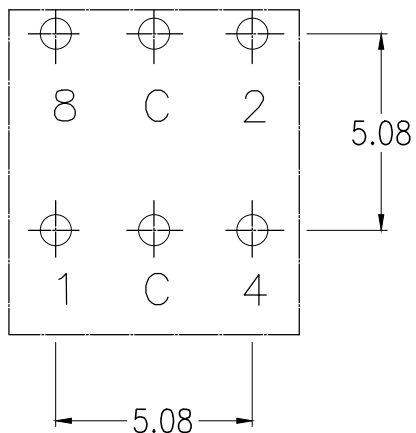
P.C.B. DIMENSION
