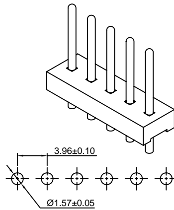
P.C.B LAYOUT
