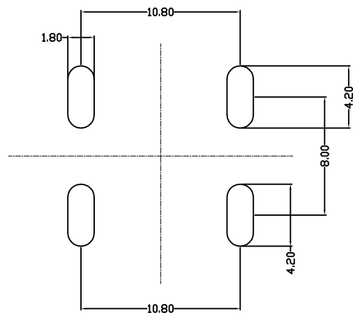
PCB插板参考尺寸
