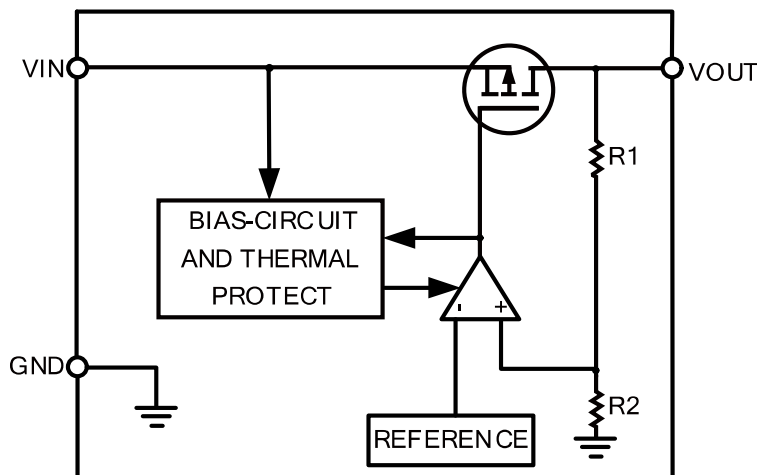
功能框图
