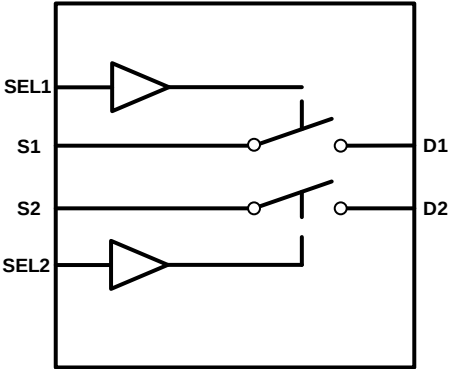
RS2266 功能框图
