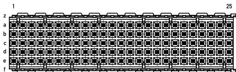
■ = bestückt / assemble
