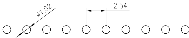
P.C.B LAYOUT
