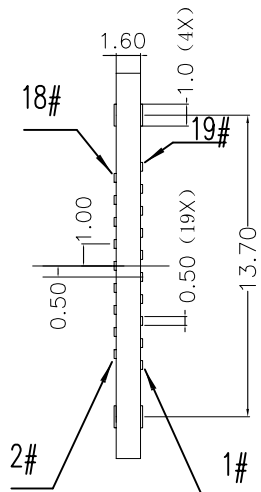
P.C.B LAYOUT
