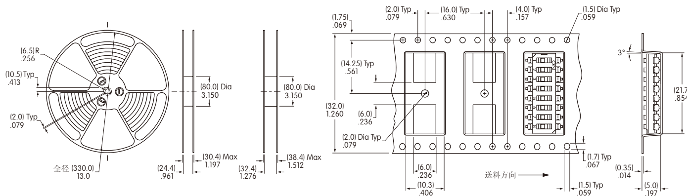
盘尺寸 JSO204AP4-R JSO208AP4-R
