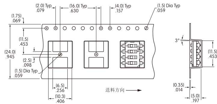
用于JSO204AP4-R的磁带尺寸
