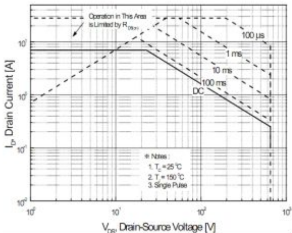
图 6-1 DM7N65C(TO-220) 最大安全工作区曲线 Fig6-1 Maximum Safe Operating Area
