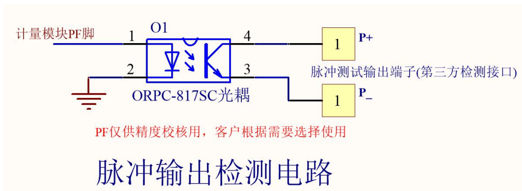
IM1281B 脉冲检测接口接线示意图
