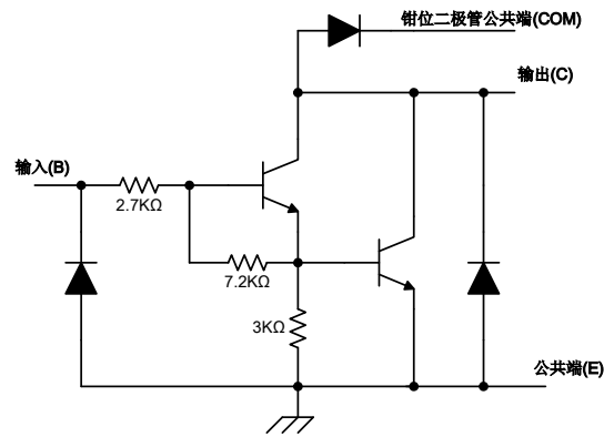
ULN2802 单路驱动电路原理图
