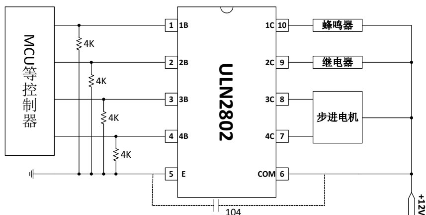
图 10 ULN2802 应用示意图
