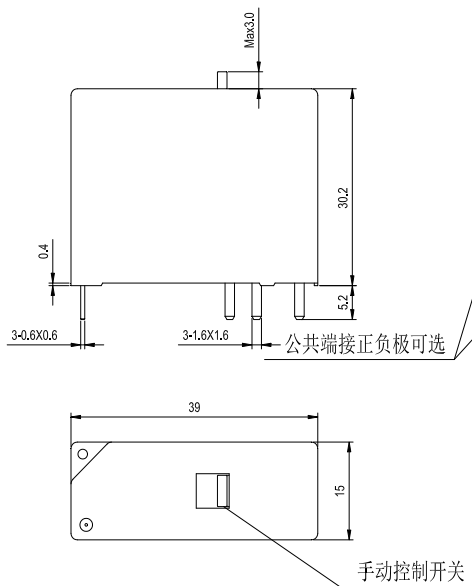
外形尺寸图
