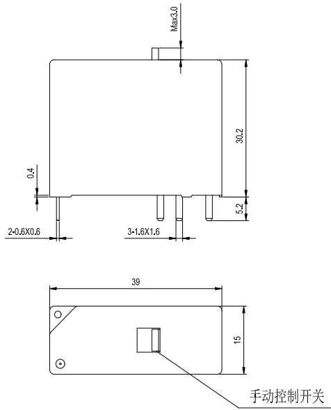
外形尺寸图
