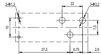
安装尺寸图
