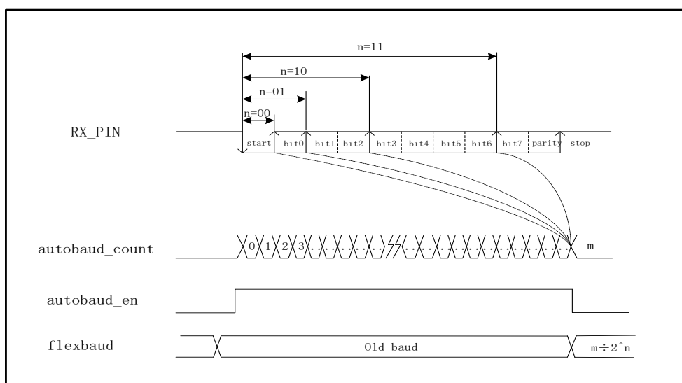
图 6-28 自动波特率示意图
