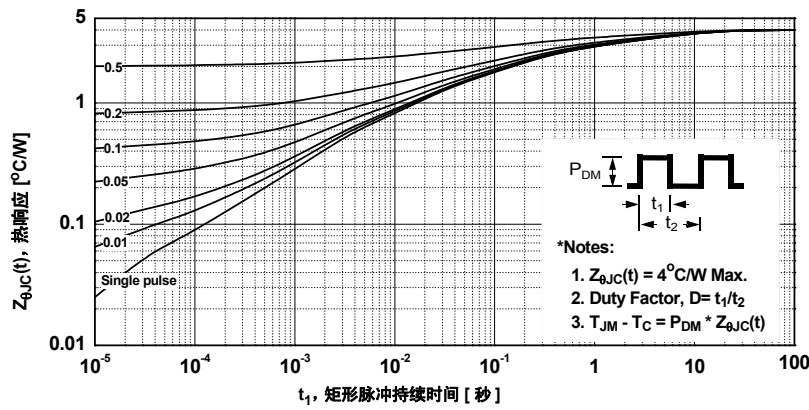
图 14. 瞬态热响应曲线 (FCPF380N60)
