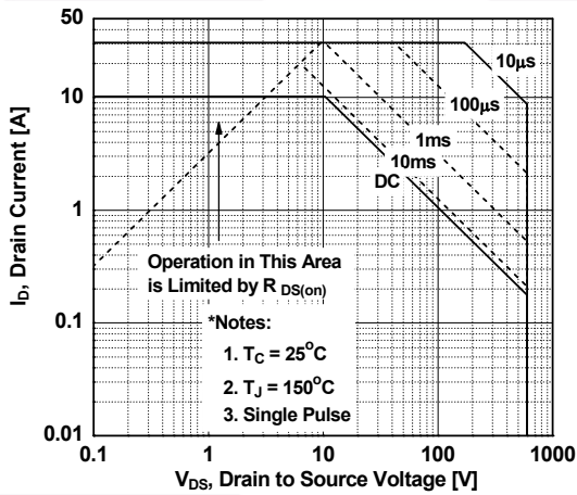
图 9. 最大安全工作区 (FCP380N60)
