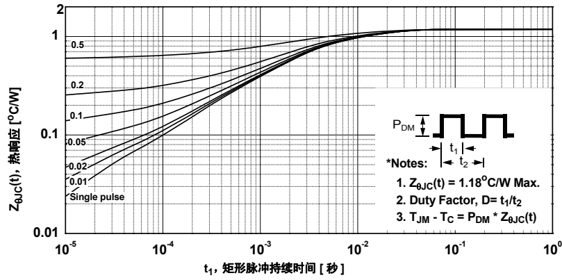
图 13. 瞬态热响应曲线 (FCP380N60)
