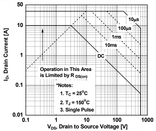
图 10. 最大安全操作区 (FCPF380N60)
