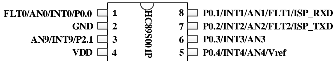
Figure 1-2 SOP8 引脚配置图
