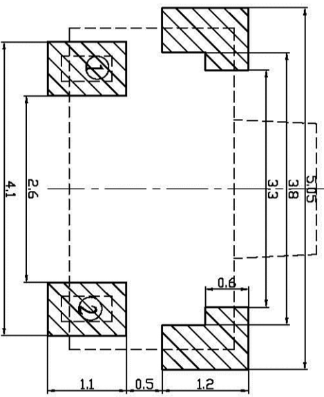
安装参考图
