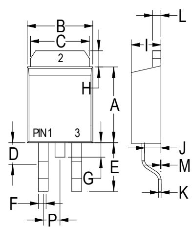
TO-263
