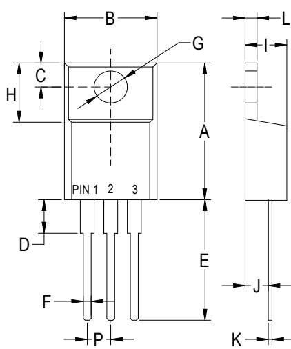
ITO-220AB
