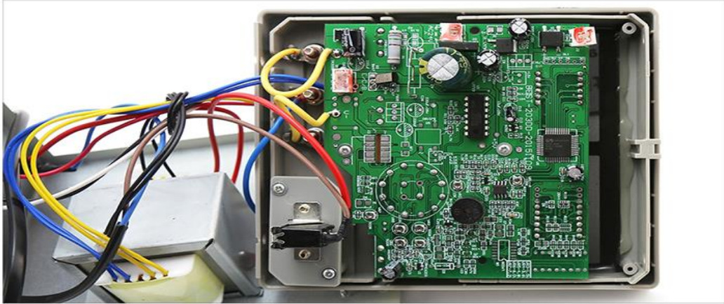
▲ PCB集成主板 双面贴片技术
