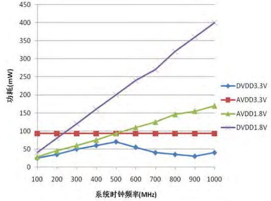
图 12 功耗与系统时钟的关系 (PLL 禁用)
