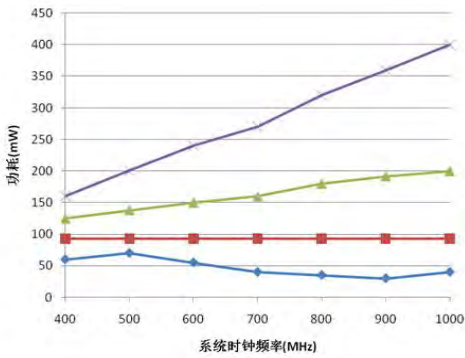
图 13 功耗与系统时钟的关系 (PLL 使能)
