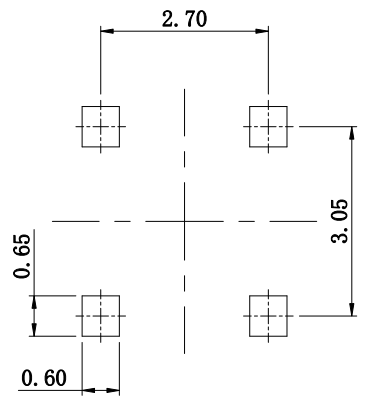
印刷板安装孔图 P.C.B Mounting pattern dimension
