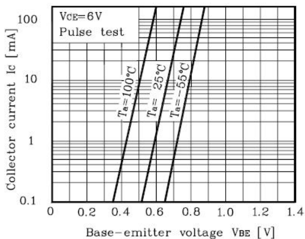
Fig. 2 I_C - V_{BE}
