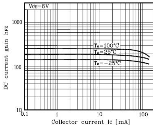
Fig. 6 h_{FE} - I_C
