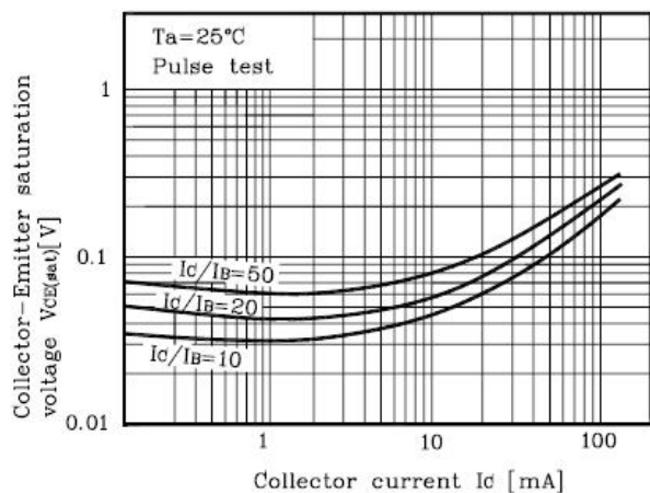
Fig. 5 V_{CE(sat)} - I_C
