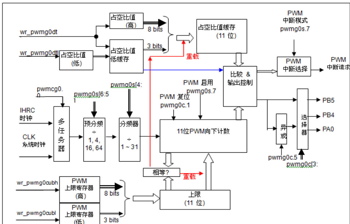
图 17: 11 位 PWM 生成器 (PWMG0) 硬件框图
